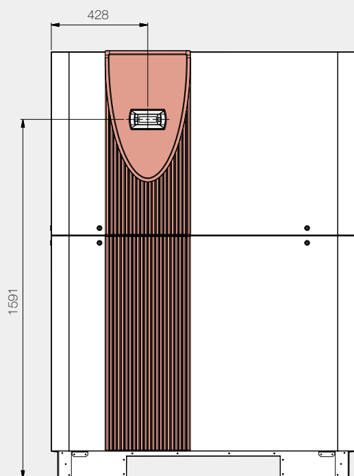
Rysunek wymiarowy
