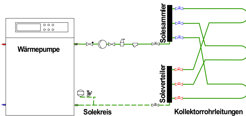
Abb. 1.1: Wärmepumpenkreislauf Wärmequellenseite
